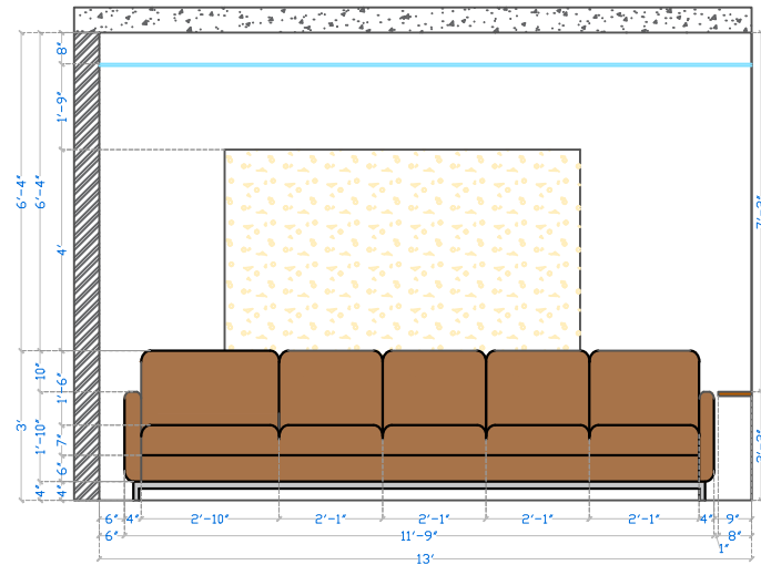
ELEVATION B
