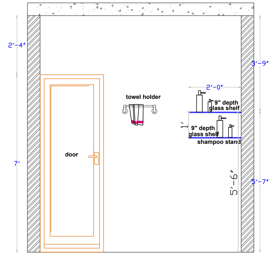
ELEVATION B
