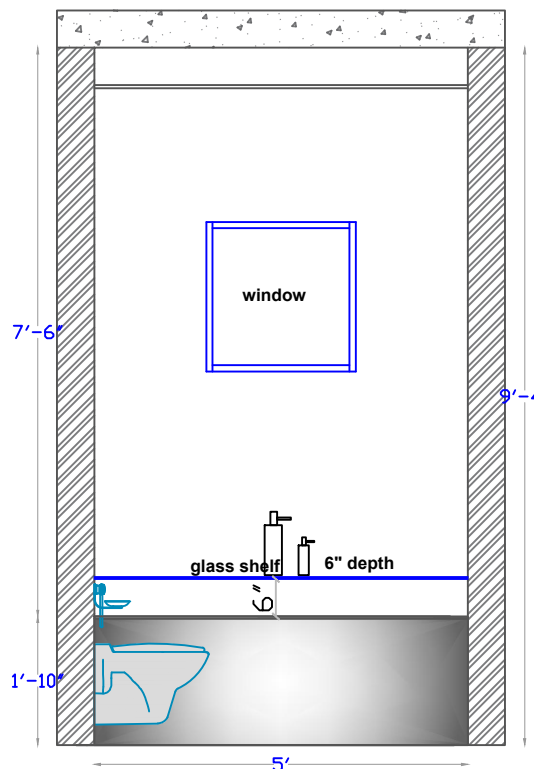
ELEVATION B
