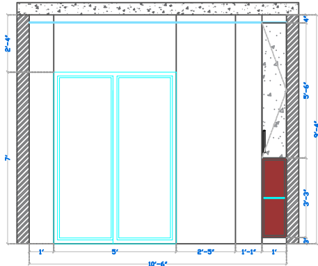
ELEVATION A
